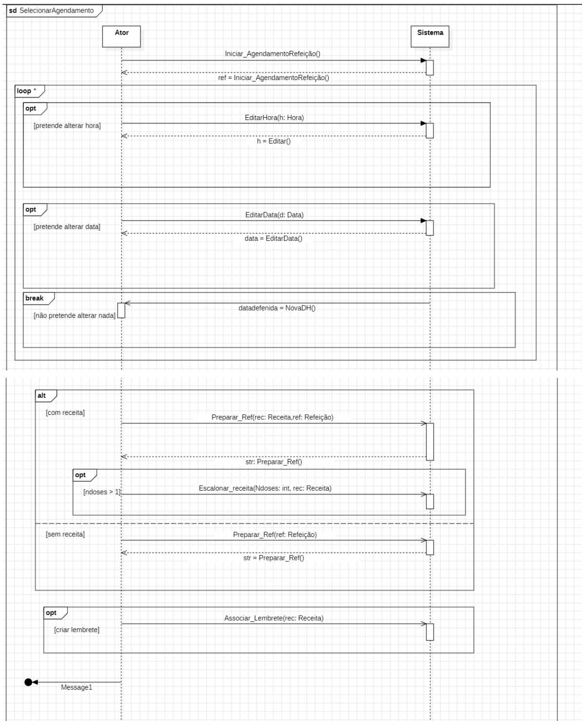
Figura 2 - Diagrama de Sequência do Sistema
