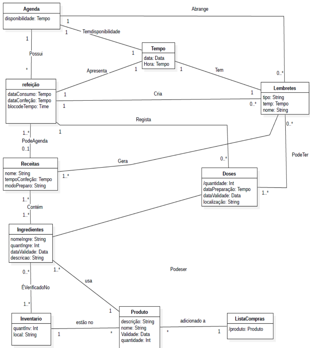
Figura 1 - Modelo de Domínio
